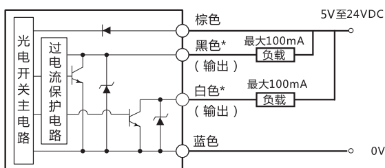
NPN
