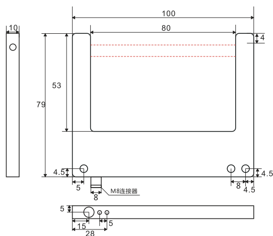
UC-SPM80(D)N-M1
