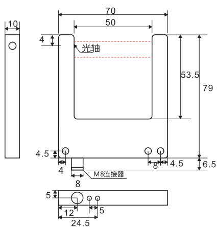
UC-SPM50(D)N-M1
