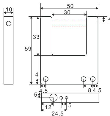
UC-SPM30(D)N-M1
