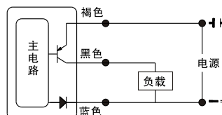
无触点PNP/常开型
