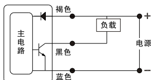
无触点NPN/常开型
