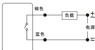
无触点NPN/常开型
